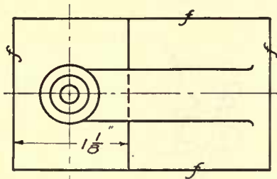
BASE C.Iron.
